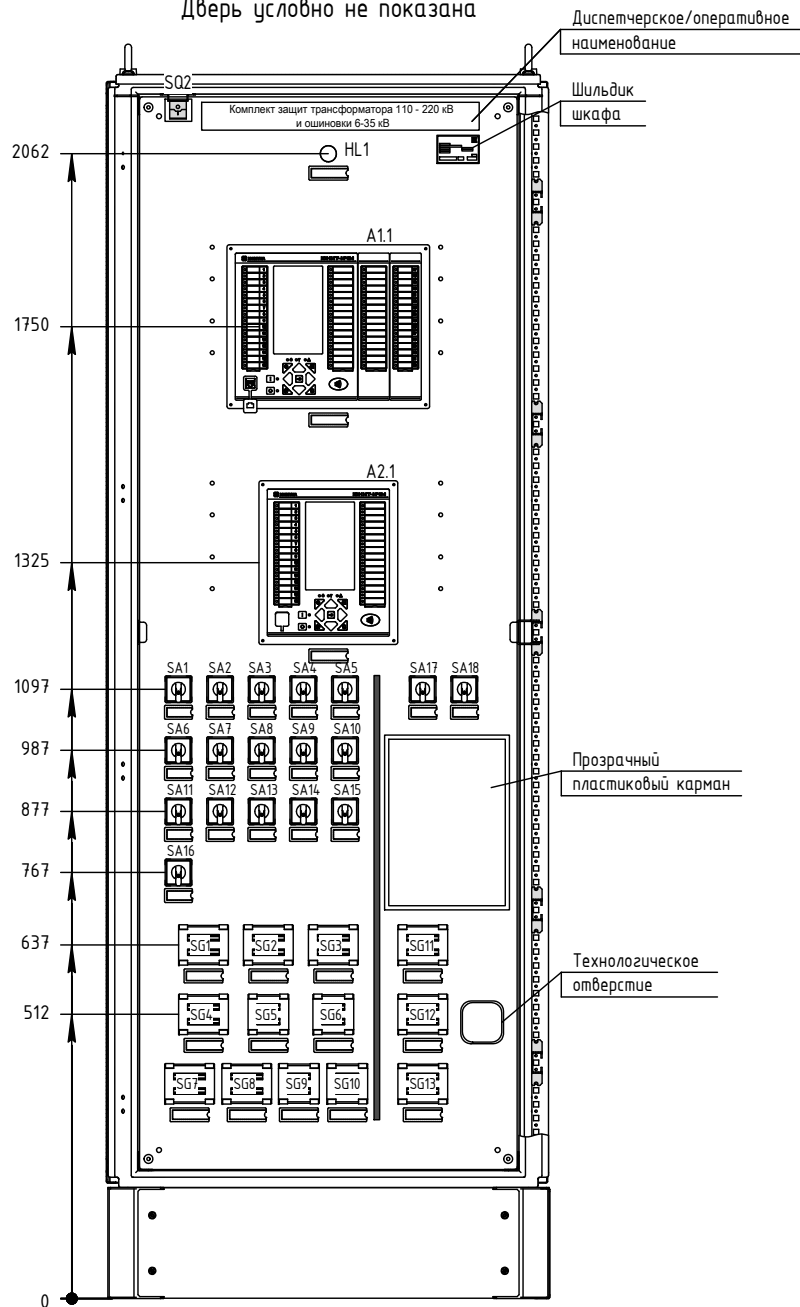
Вид спереди Дверь условно не показана
